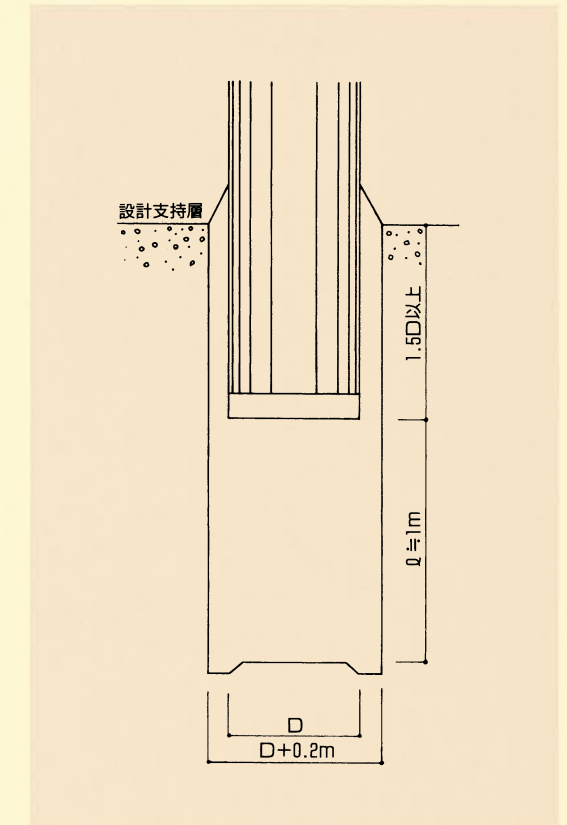
杭先端付近状況図
