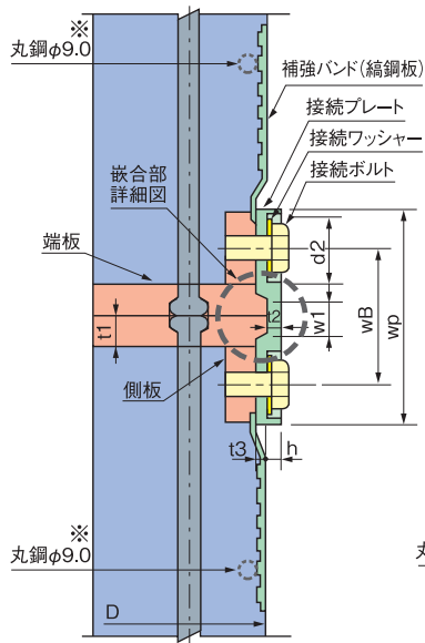
PHC杭+PHC杭の例
