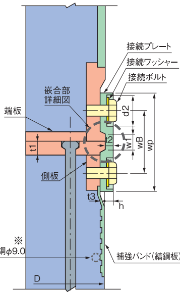
PHC杭+SC杭の例
